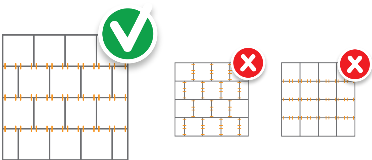
Goed halfsteensverband
